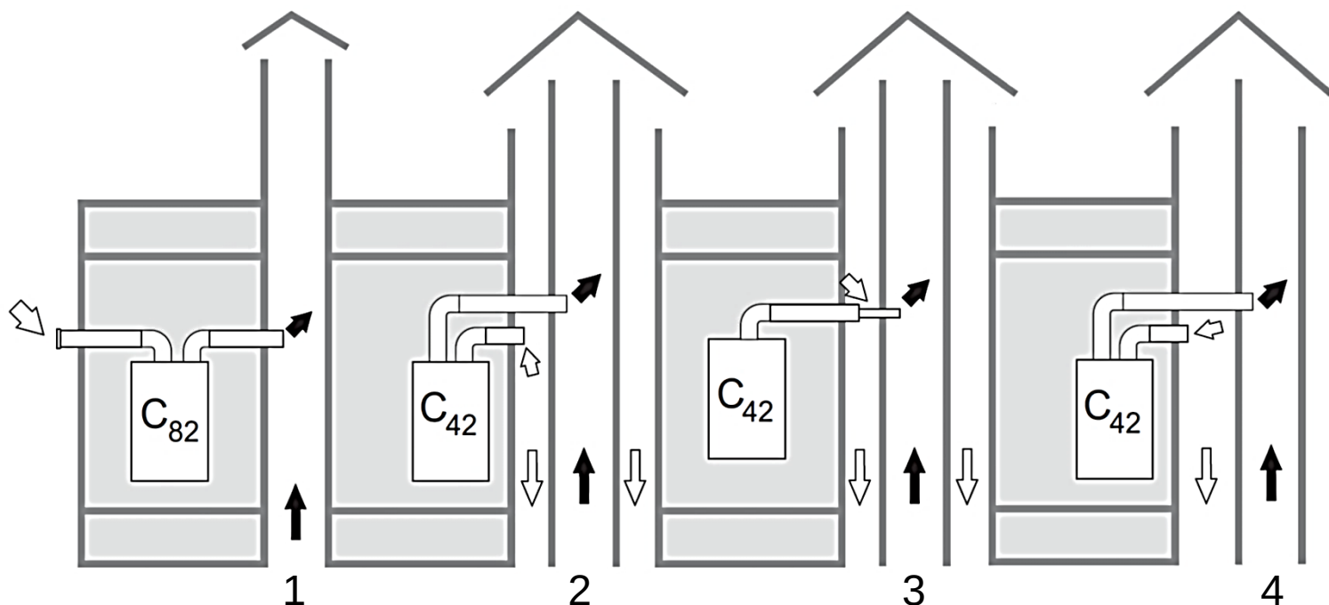
Рис. 36 Общедомовые (коллективные) системы дымоудаления.
