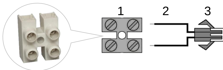
Рис. 45 Подключение клеммной колодки к разрезанной перемычке.
