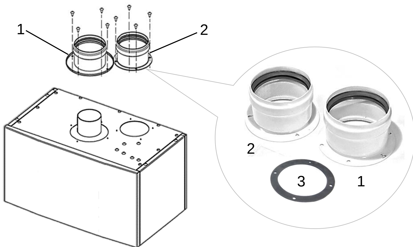
Рис. 33 Установка присоединительных фланцевых элементов для подключения раздельной системы дымоудаления Ø 80x80 мм
