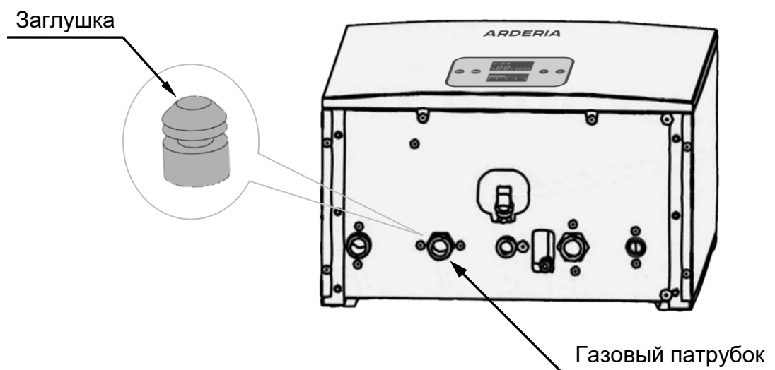
Рис. 18 Место присоединение котла к газопроводу
