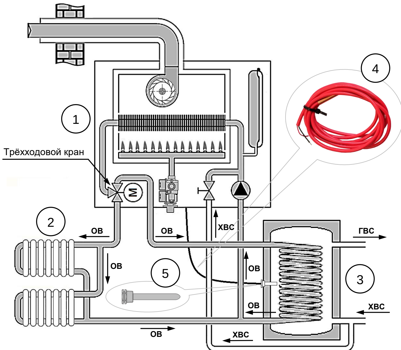
Рис. 24 Принципиальная монтажная схема подключения одноконтурного котла со встроенным трёхходовым клапаном к емкостному водонагревателю косвенного нагрева (бойлеру)
