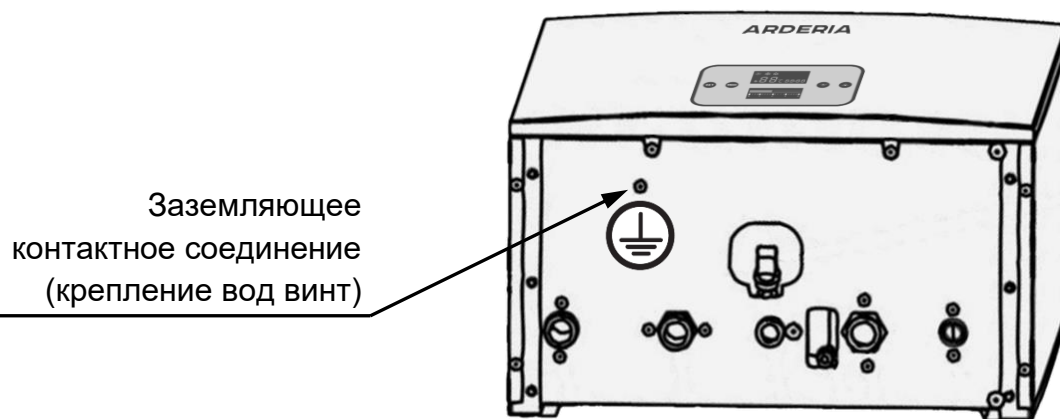
Рис. 17 Заземляющий контакт
